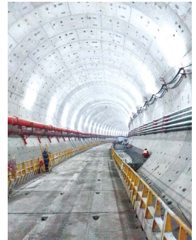
北横通道采用预制拼装工艺完成首段急曲线施工
